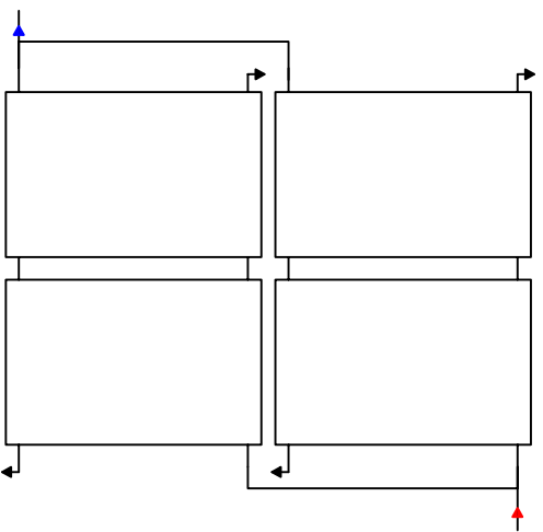
Verschaltung von 4 Kollektoren Reihe/Parallel (2 x 2er Montageset)
