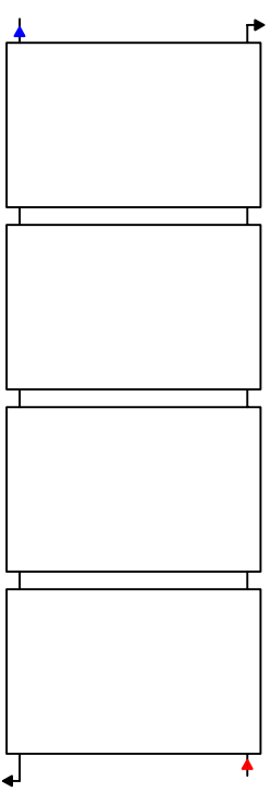
Verschaltung 4 Kollektoren in Reihe (2 x 2er Montageset)
