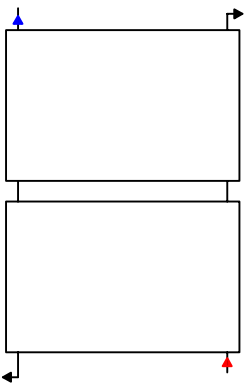
Verschaltung 2 Kollektoren (1 x 2er Montageset)
