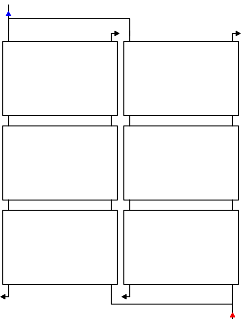
Verschaltung von 6 Kollektoren Reihe/Parallel (2 x 3er Montageset)
